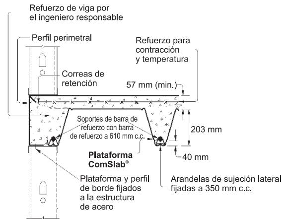
DETALLES DEL SOPORTE PERIMETRAL
