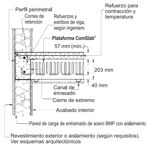
DETALLES DEL ACABADO DEL SOPORTE DE EXTREMO
