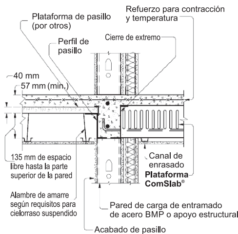
DETALLES DEL ACABADO DE PASILLO
