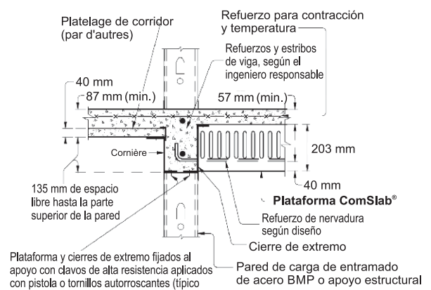
DETALLES DEL SOPORTE DE PASILLO
