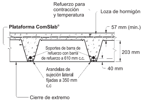
DETALLES DEL CIERRE DE EXTREMO
