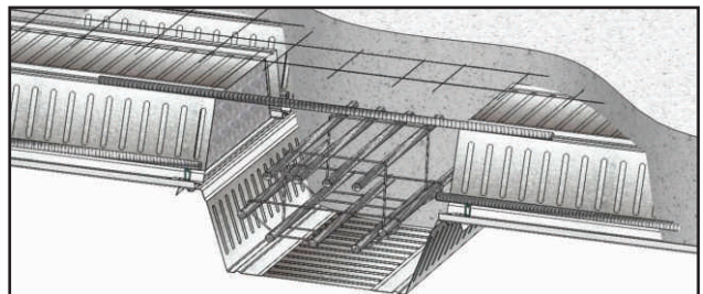
Poutre inversée ComSlab®
