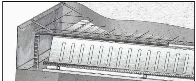
Mur extérieur en béton à coffrages isolants
